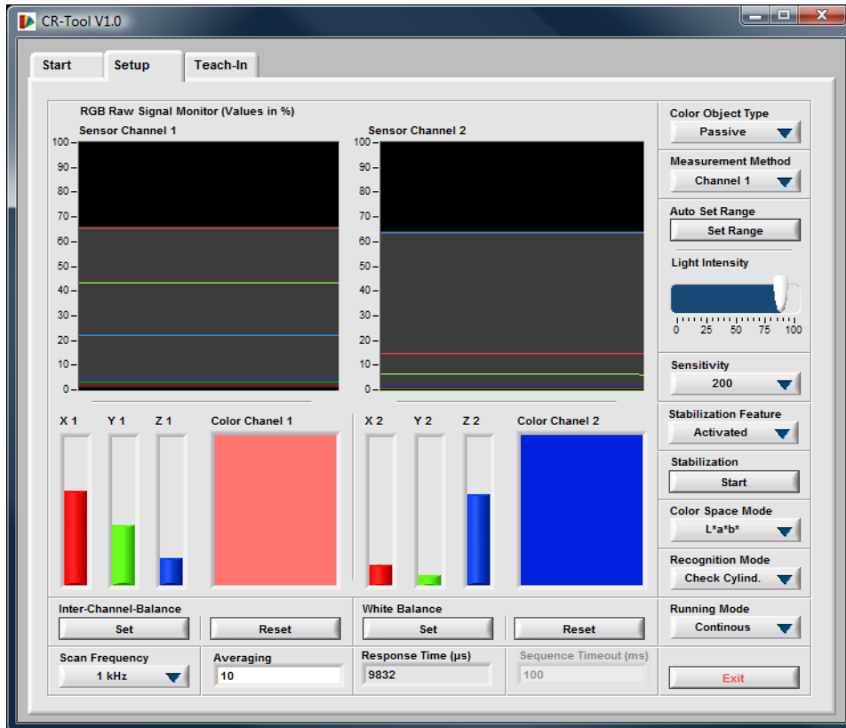
Fig. 4 Parameter setup tab
